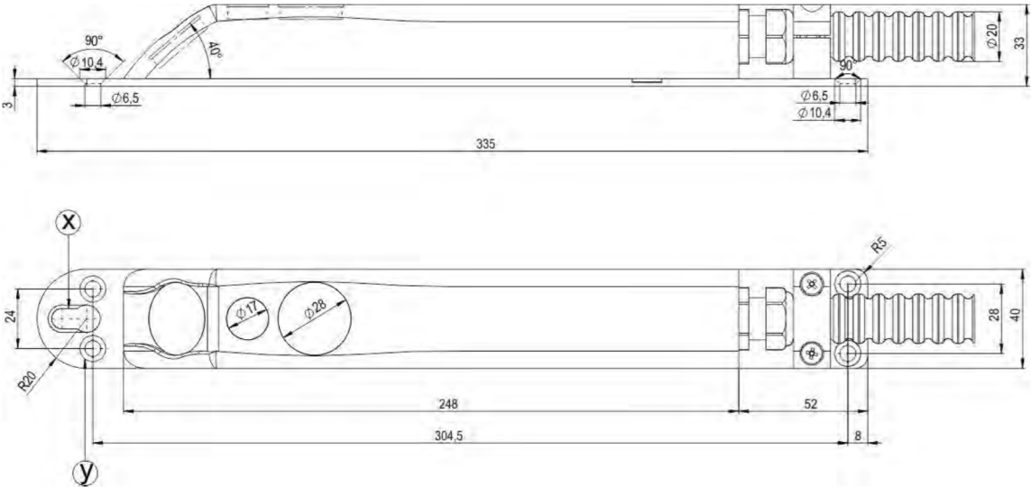
Fig. 4-23 Dimensions sensor CS2-....K
