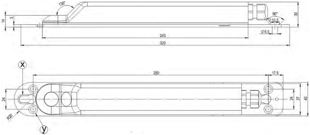
Fig. 4-16 Dimensions sensor POA-V2H1K / POA-V2U1K
